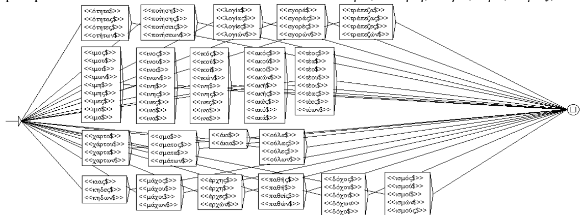
Figure 3 : Graphe de suffixes nominaux pour l'extraction des termes candidats
