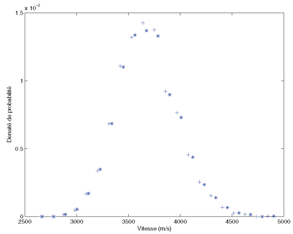
Fig. 3. Les densités de probabilité des variables aléatoires C_P (symbole *) et V (symbole +) en fonction des réalisations lorsque \alpha = 0 .
