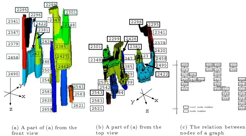
図 13 3D グラフの情報を用いて虫食い領域を分岐ごとに可視化した例 The example which visualized the gallery regions for every branch using the information on graph
