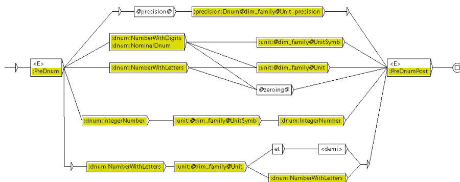
Fig. 6. parameterized SimpleDnumUnit
